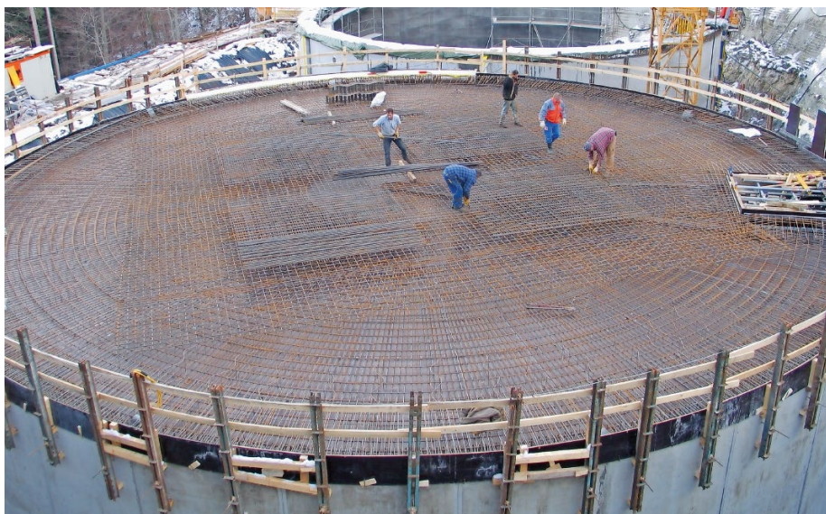
Der Brillenwasserbehälter Feldkirch, Vorarlberg, ist ein charakteristisches Siedlungswasserbau-Projekt und wurde von einem Baumeister geplant.
